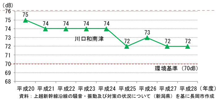
上越新幹線鉄道騒音の経年推移
