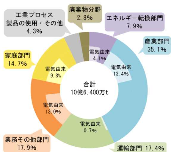
【日本の部門別CO 2 排出量（2021年度）】
