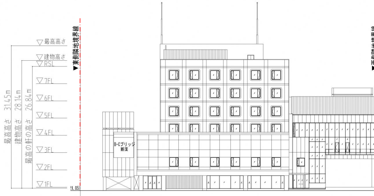
北立面図
