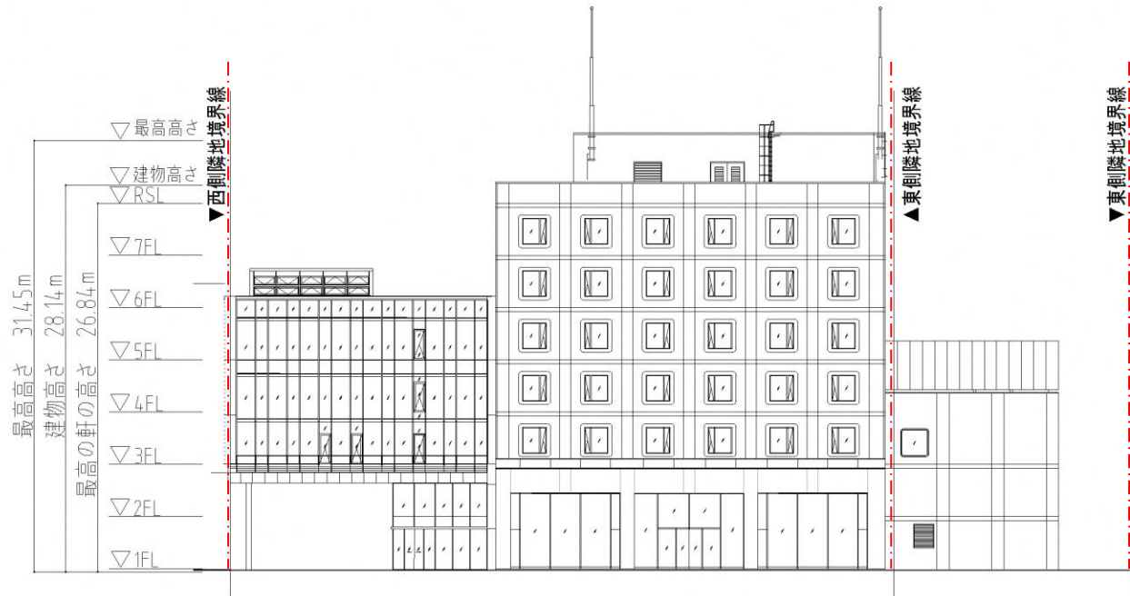
南立面図
