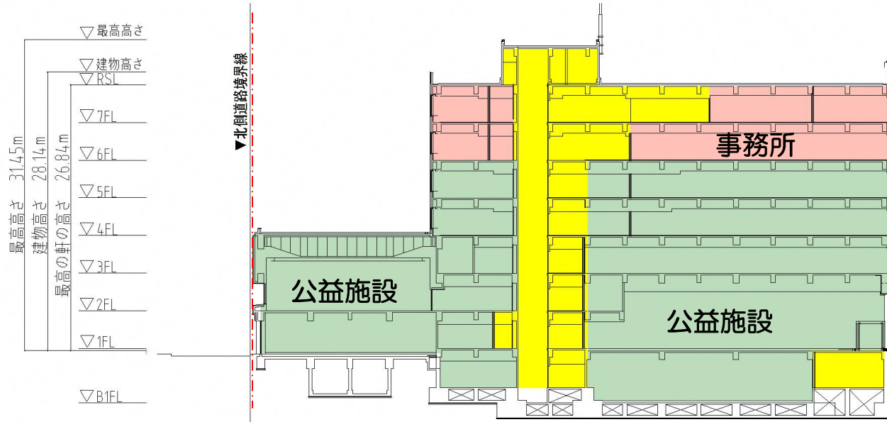
南北断面図
