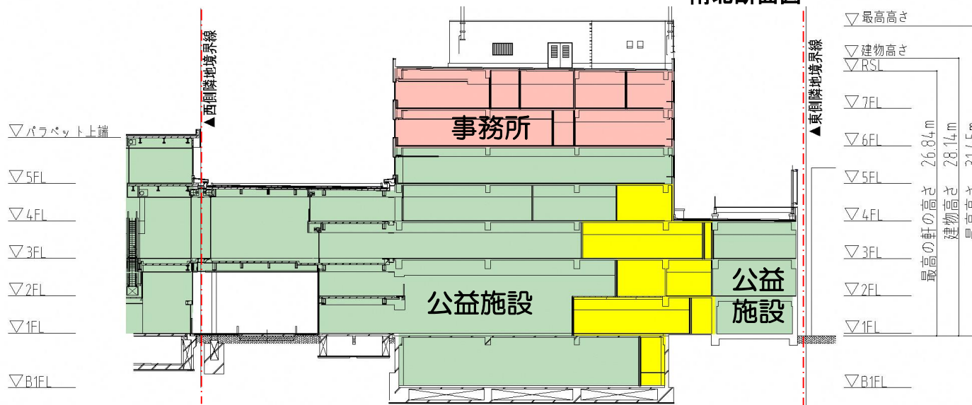
東西断面図
