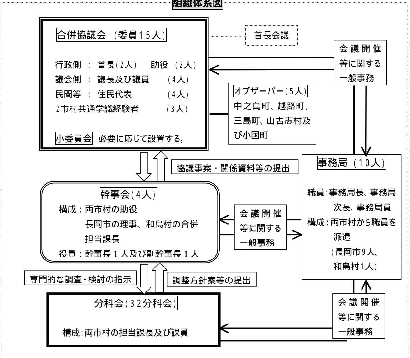
組織体系図
